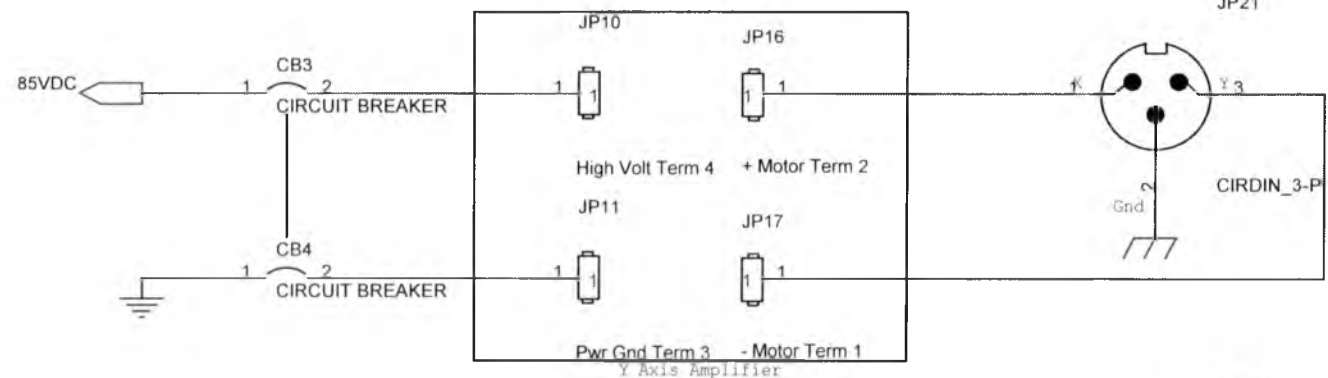
Y Axis Amplifier
